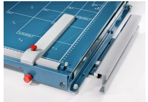
Herausziehbarer Vorderanschlag bis 170 mm mit ausklappbaren Papierhaltern - zum Schneiden von Streifen gleicher Schnittbreite
